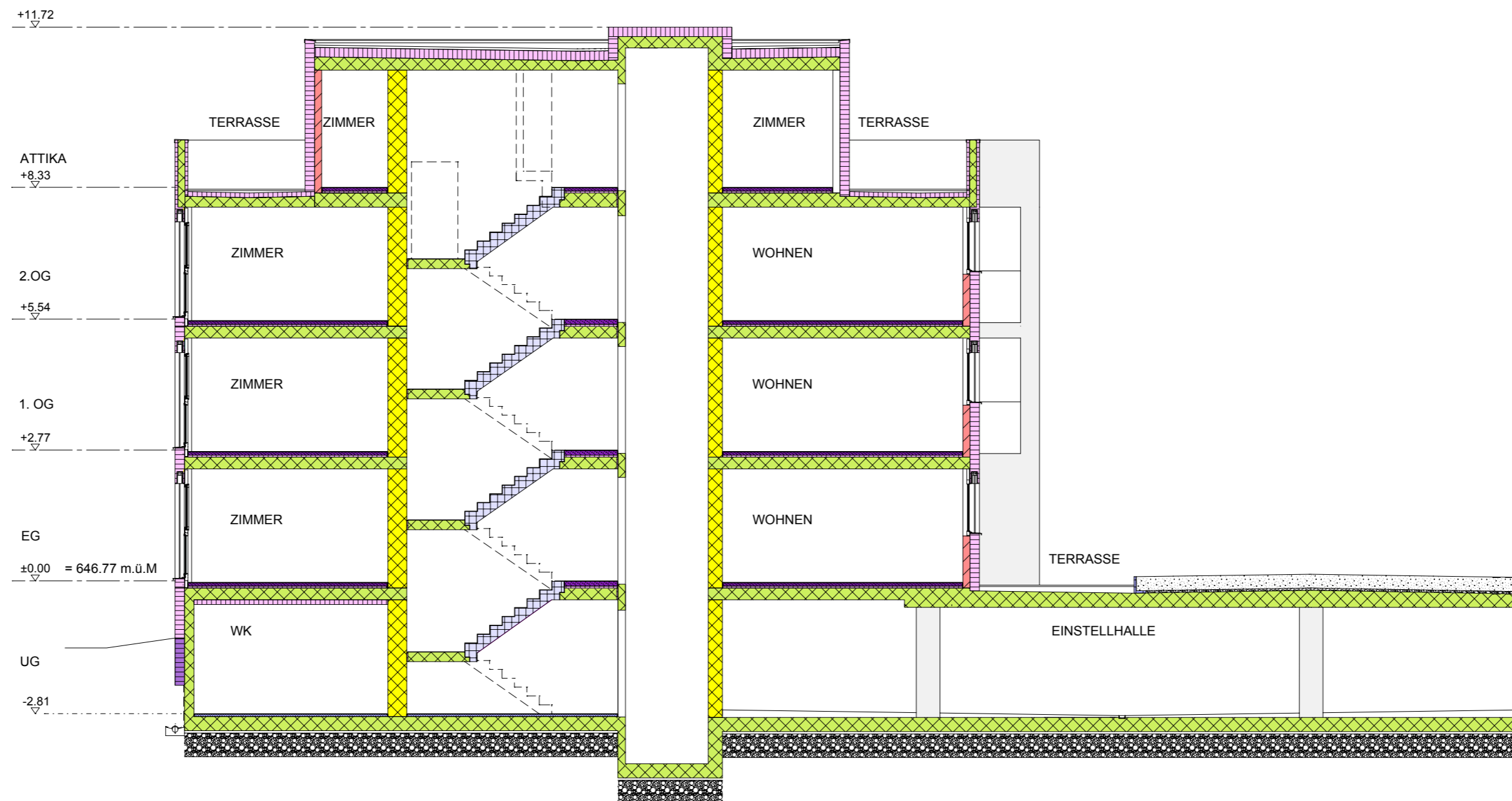
SCHNITT
